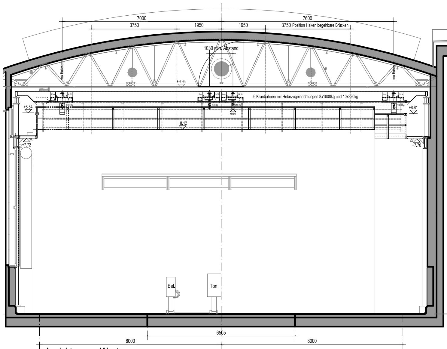
Ansicht gegen Westen
