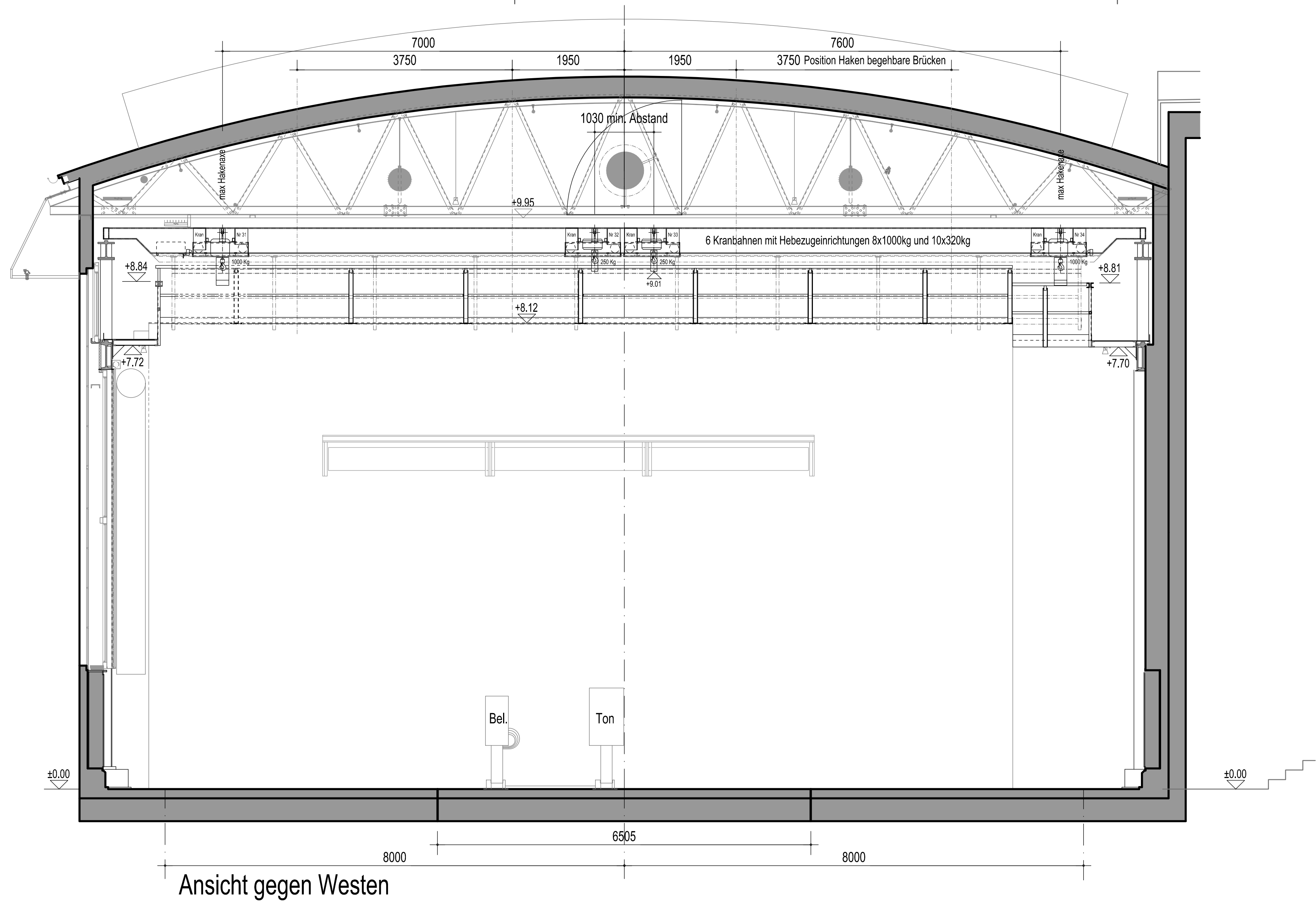
Ansicht gegen Westen
