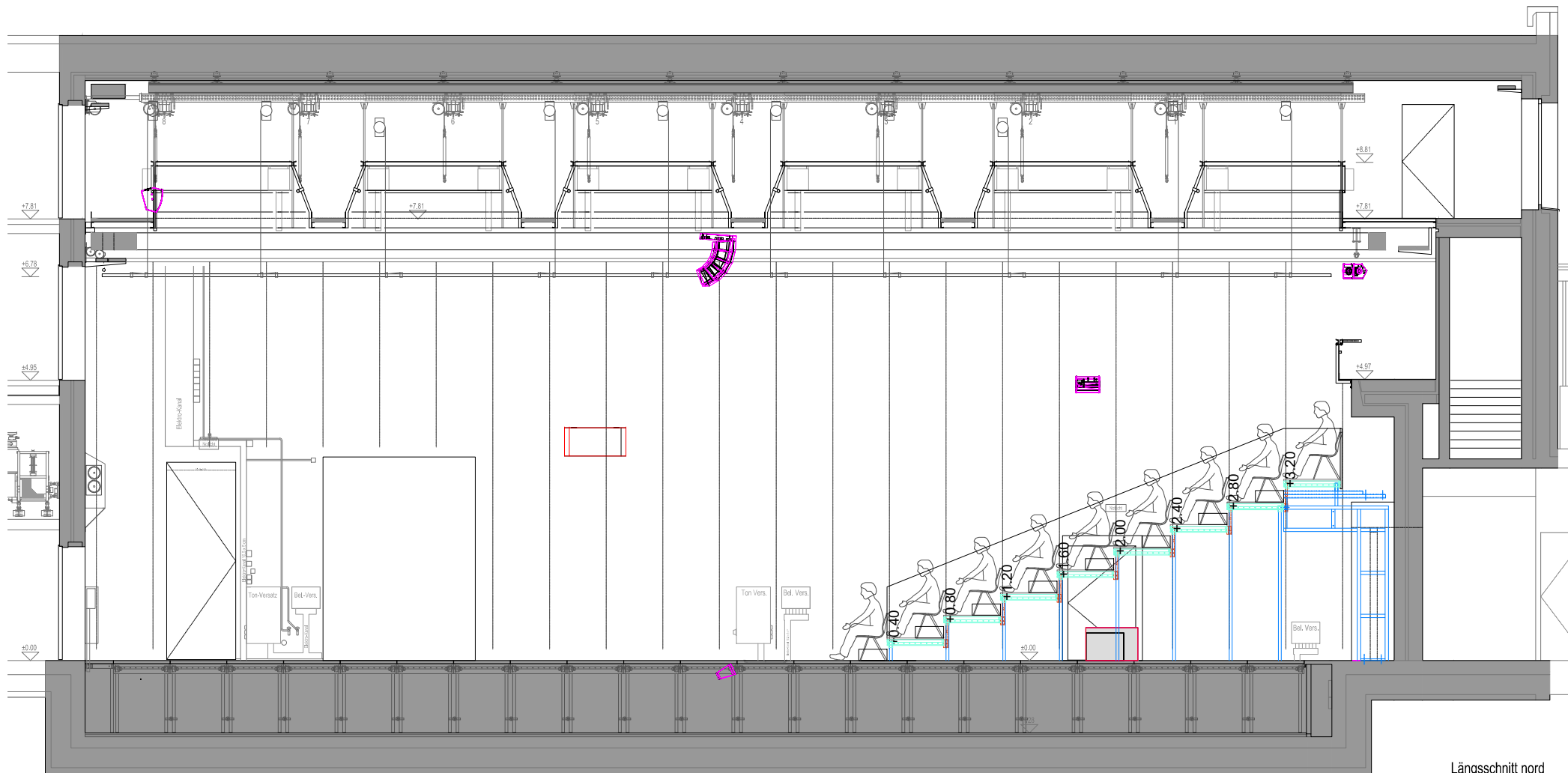
Längsschnitt nord
